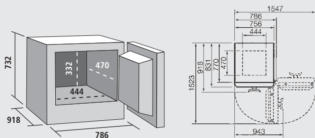
Volumen: 71 l (Maße in mm)
